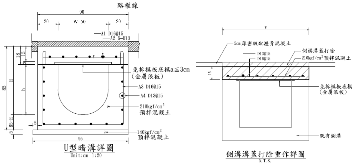
側溝設計断面參考圖說 1
