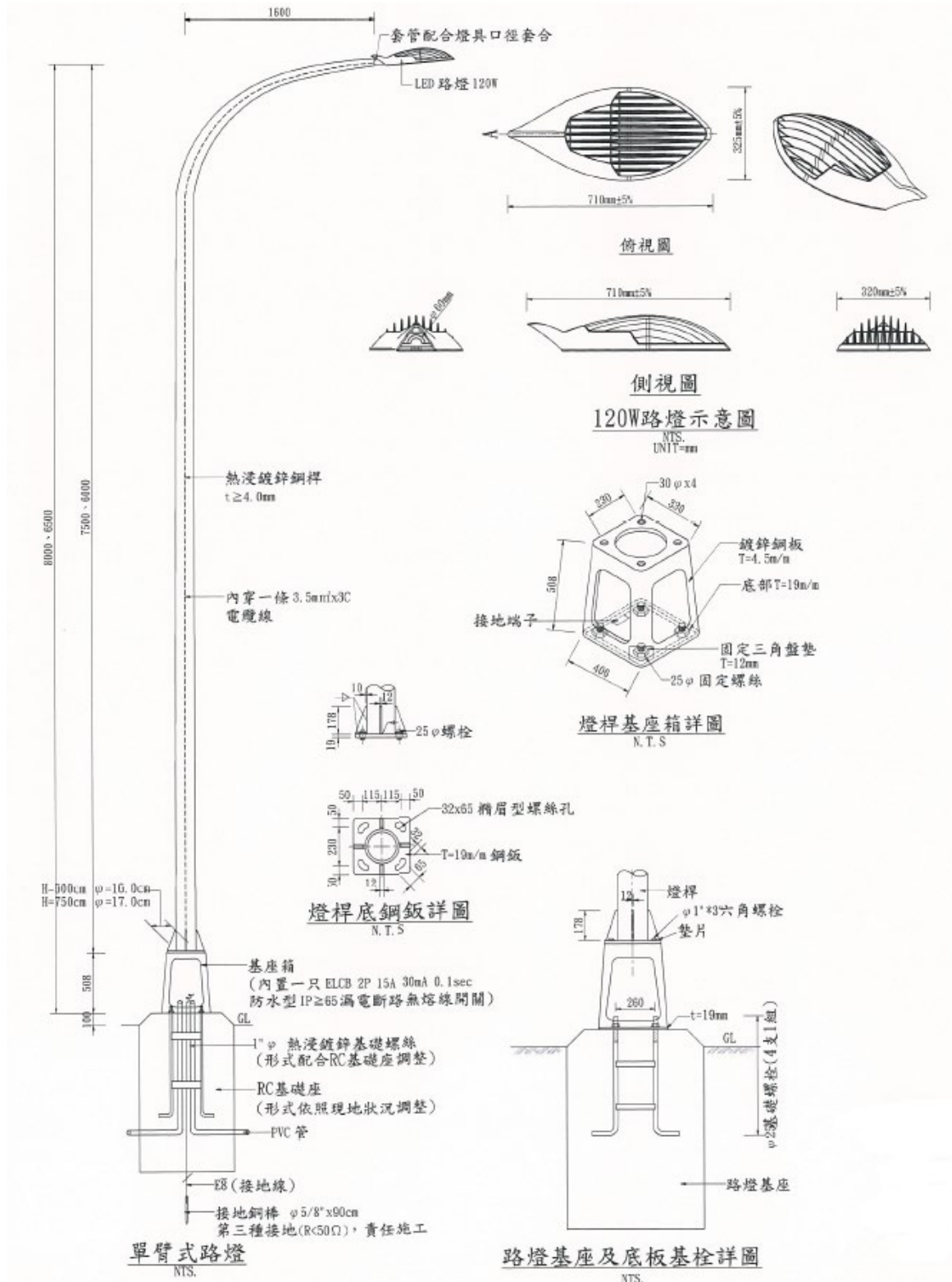
道路照明設計断面參考圖說 1
