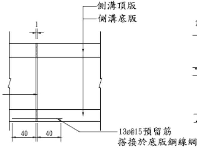
伸縮縫預留筋詳圖
