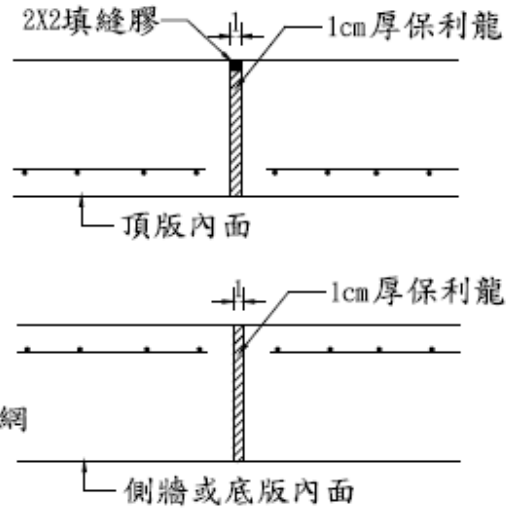
伸縮縫詳圖
