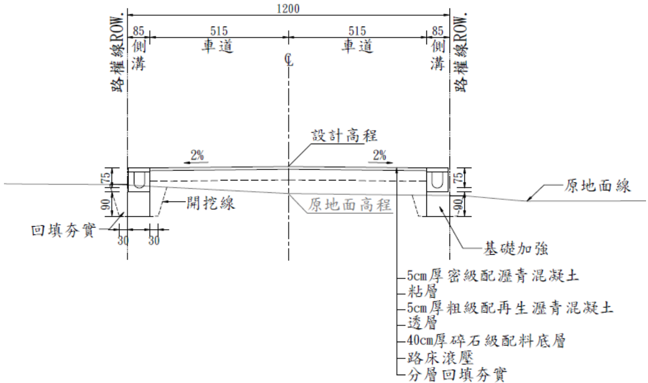
12M 道路設計断面參考圖說 1
