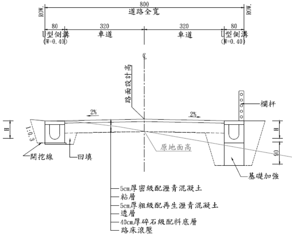
8M 道路設計斷面參考圖說 1
