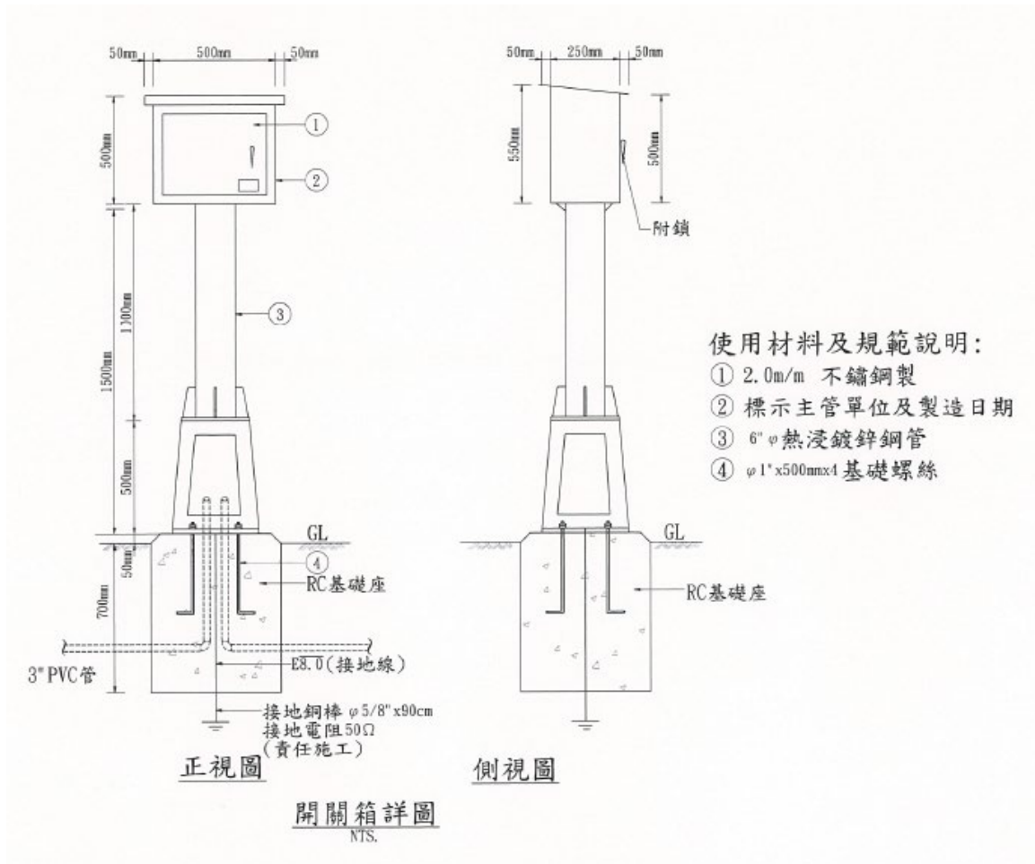
道路照明設計斷面參考圖說 2
