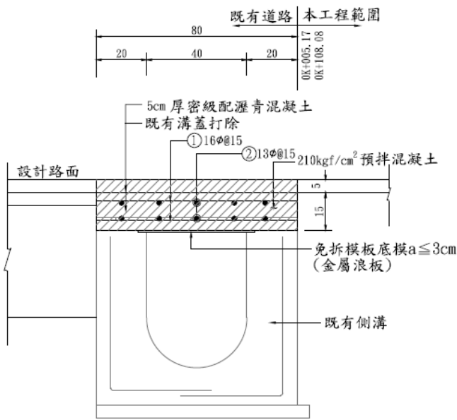
既有溝蓋打除重作詳圖
