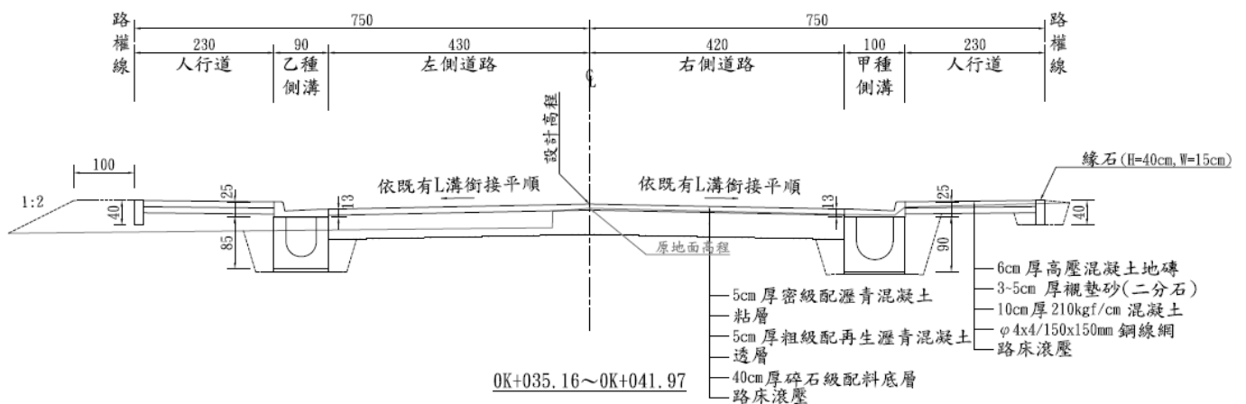
(含人行空間)道路設計断面參考圖說 1
