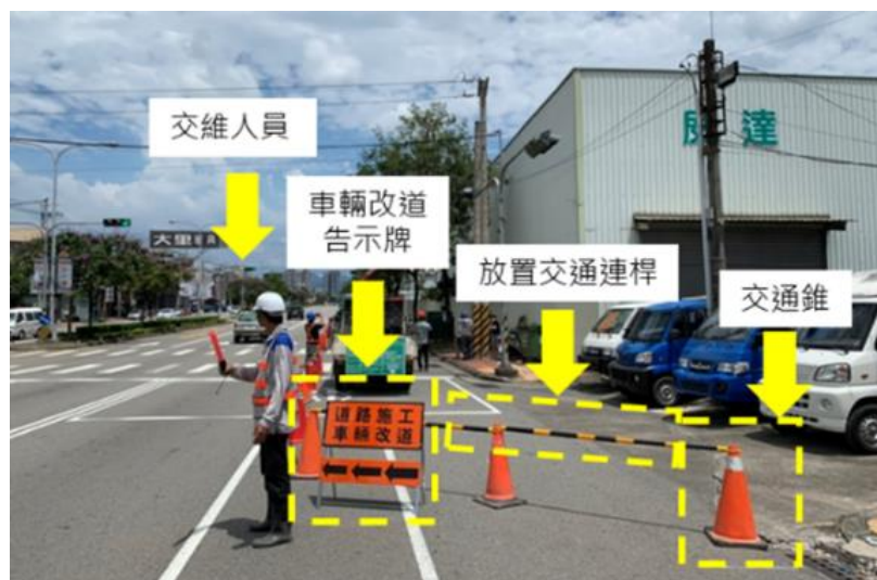
圖 7 交維布設作業圖
